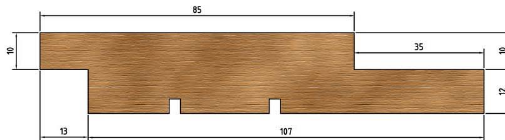
22x120 Falsad spårpanel (2525)
