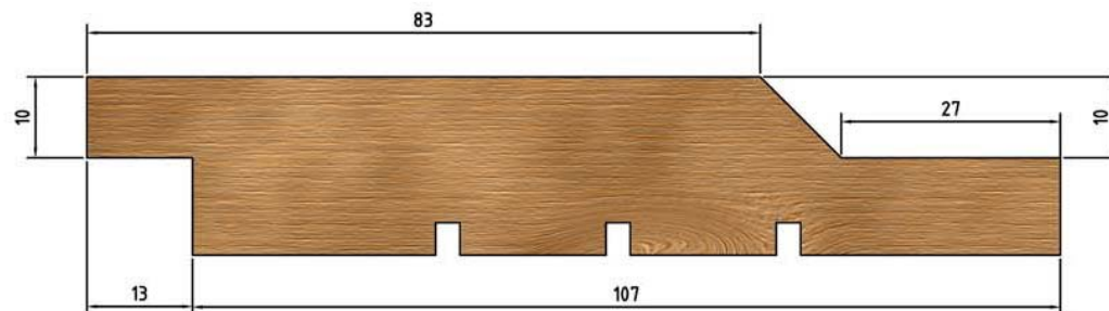
22x120 Falsad spårpanel med fasad kant (2515)
